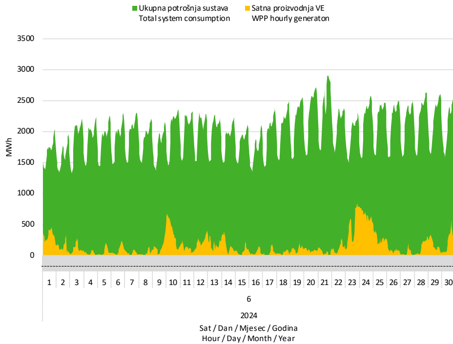
Slika 7 Usporedba satnog dijagrama opterećenja sustava i proizvodnje vjetroelektrana u lipnju 2024. godine
