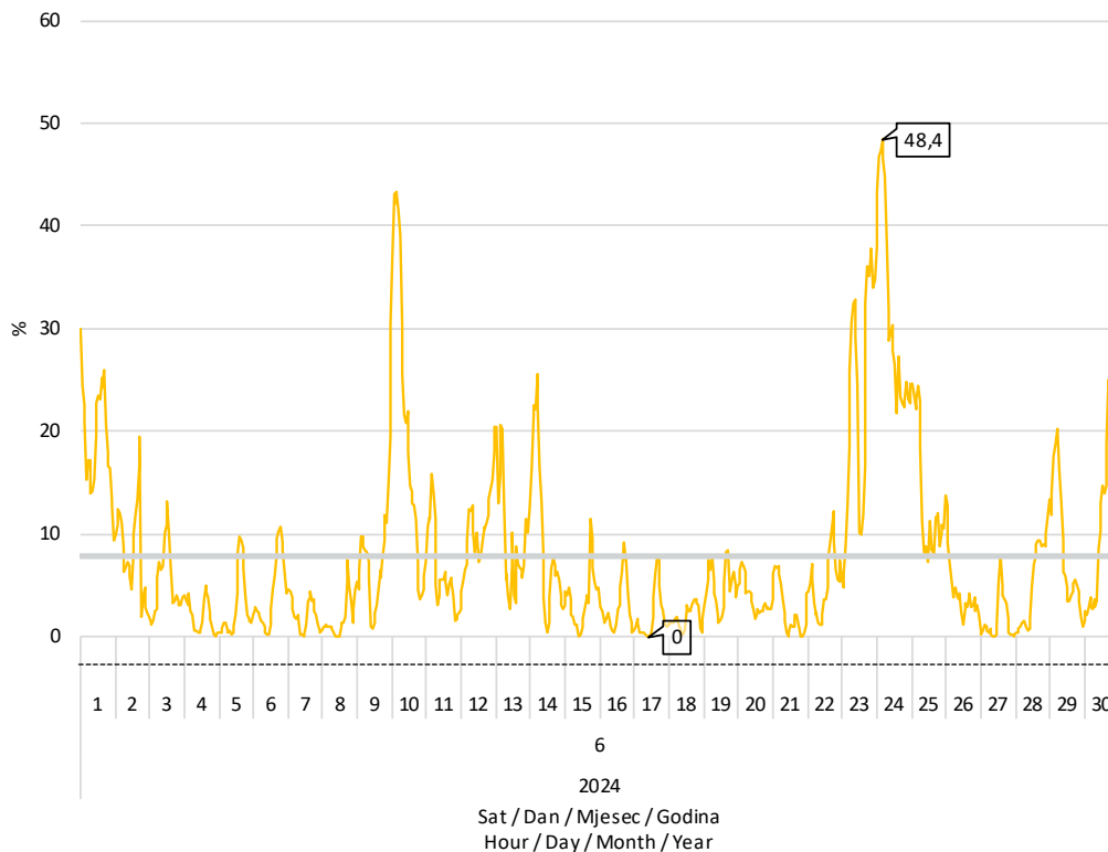
Slika 8 Udio proizvodnje vjetroelektrana u pokrivanju satnog opterećenja elektroenergetskog sustava u lipnju 2024. godine
