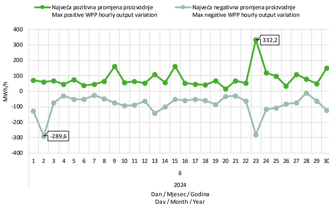
Slika 9 Maksimalna pozitivna i maksimalna negativna promjena satne proizvodnje VE u lipnju 2024. godine
