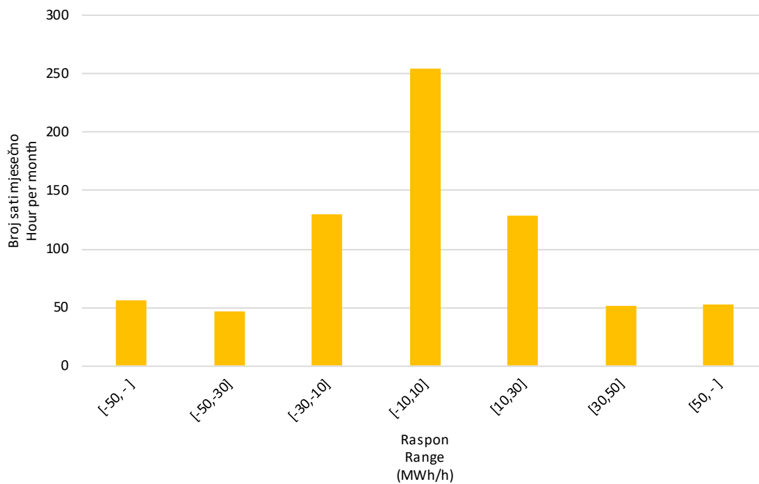
Slika 10 Statistička raspodjela satnih promjena proizvodnje VE u lipnju 2024. godine
