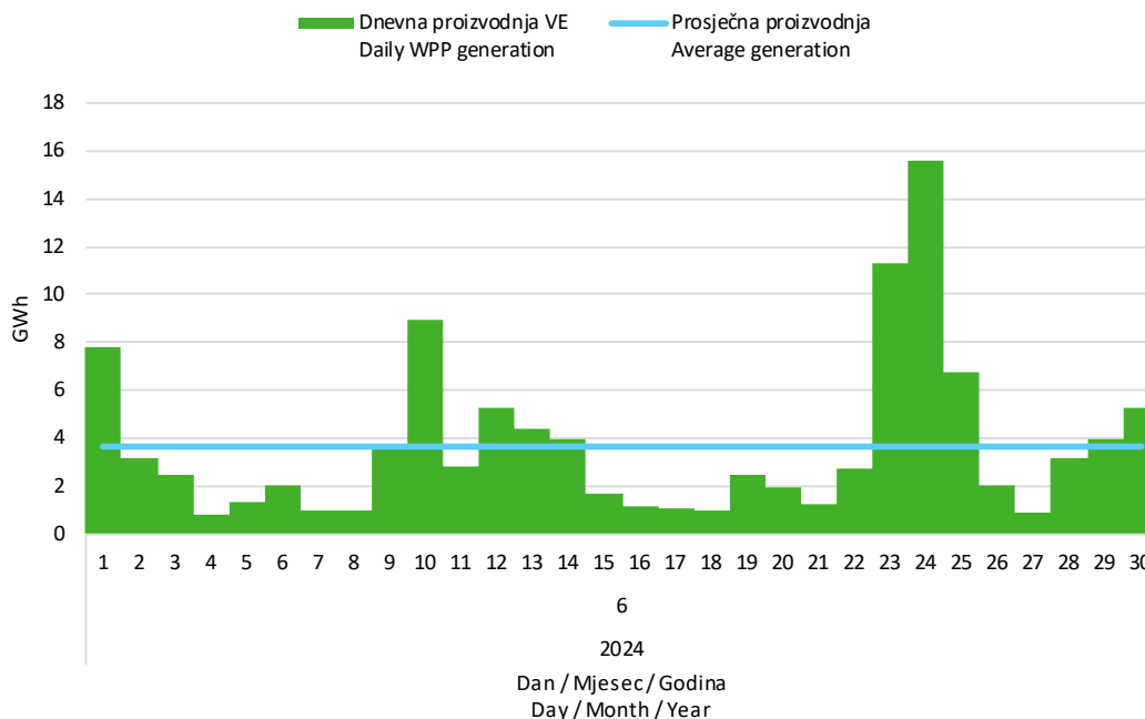
Slika 5 Dnevna proizvodnja svih vjetroelektrana u lipnju 2024. godine
