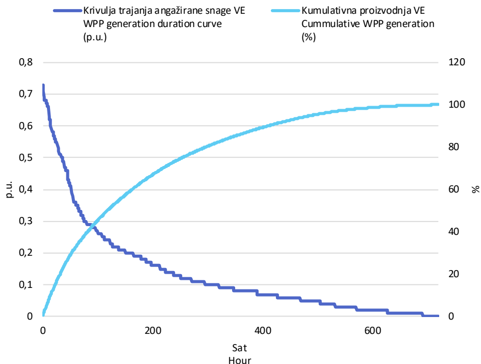
Slika 3 Krivulja trajanja angažirane snage svih VE i kumulativna proizvodnja VE u lipnju 2024. godine u jediničnim vrijednostima
