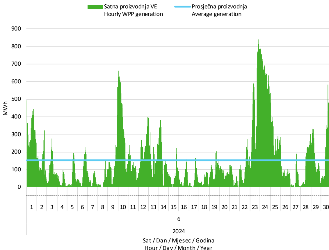
Slika 2 Satna proizvodnja svih vjetroelektrana u lipnju 2024. godine
