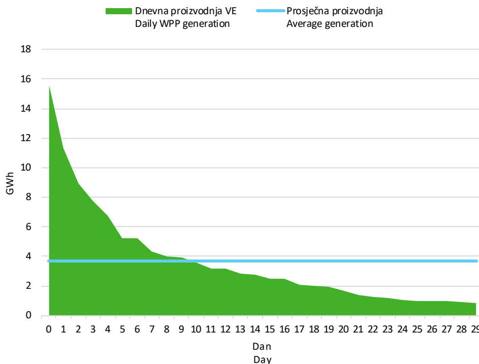
Slika 6 Krivulja trajanja dnevne proizvodnje vjetroelektrana u lipnju 2024. godine
